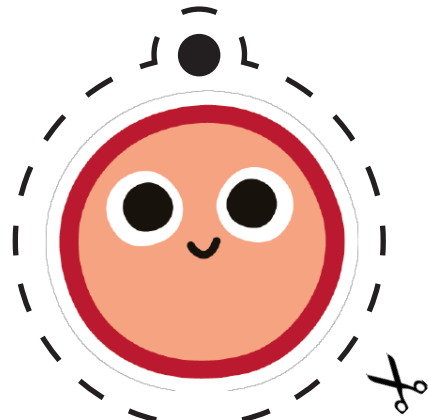
Venus
