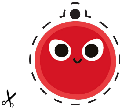
Mart
