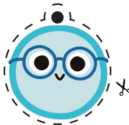
Urà
