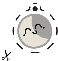
Lluna
